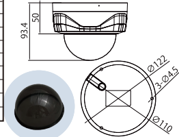
■外形寸法 (mm)
