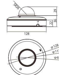
■外形寸法 (mm)
