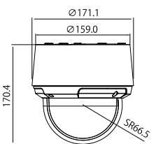
■外形寸法(mm)
