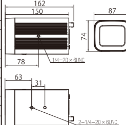
■外形寸法 (mm)
