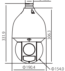
■外形寸法(mm)
